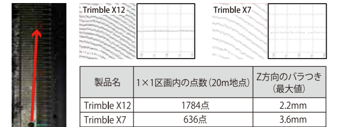
20m先に設置した1m×1mの区画内のスキャン点数とZ方向に対して精度比較を検証
