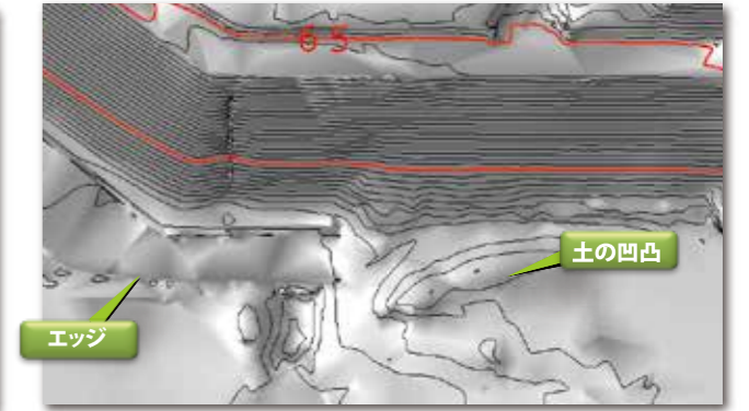
最適化後の面の一部。点群精度10cm以内で間引きたことで、土の凹凸が消え、滑らかに表現されている。小構造物などのエッジはかろうじて残っている程度。等高線を作図すると、滑らかな線図形が作成されている
