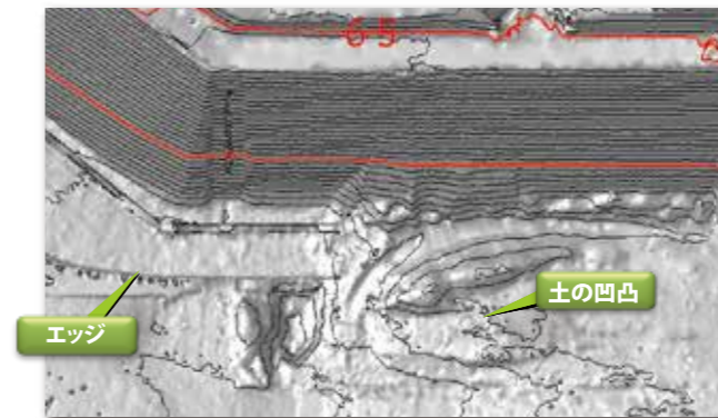
最適化前の面の一部。工事中の道路を3Dスキャナーで計測した点を面化したもの。盛り上がった土の状態や小構造物のエッジなどがリアルに表現されており、実際の形状に近い。この面を使用して等高線を作図すると、線図形が細かく波打った状態になる
