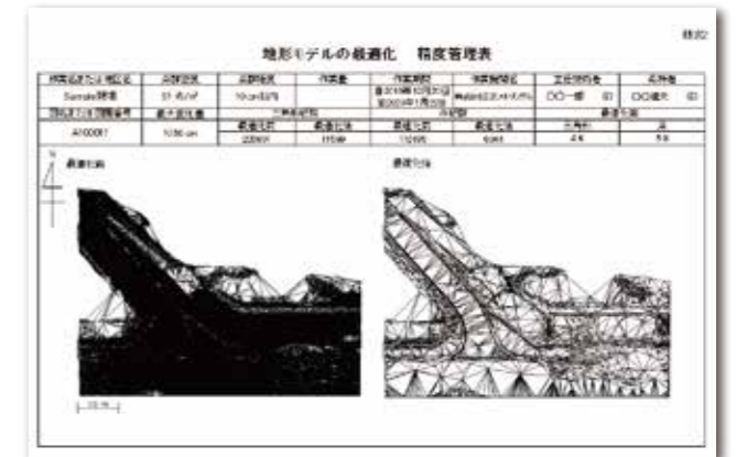
最適化を実行することで出力される精度管理表 総点数が118,195点から6,044点に減り、点数は元の5%に削減されている
